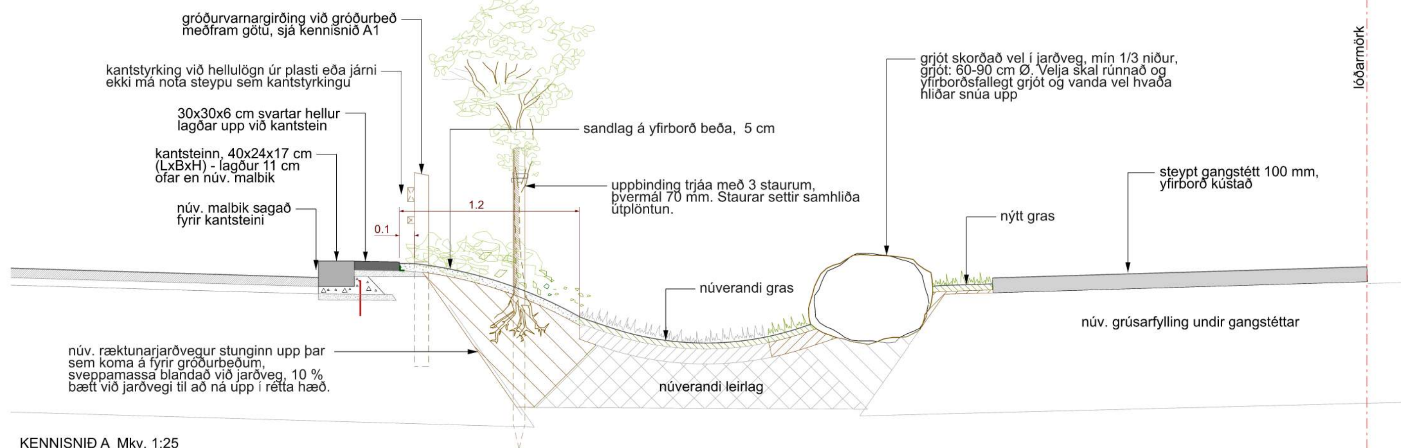
KENNISNIÐ A Mkv. 1:25 Kantur, gróðurbeði við götu og bílastæði, gróðurvarnargirðing, grjót í grasi
