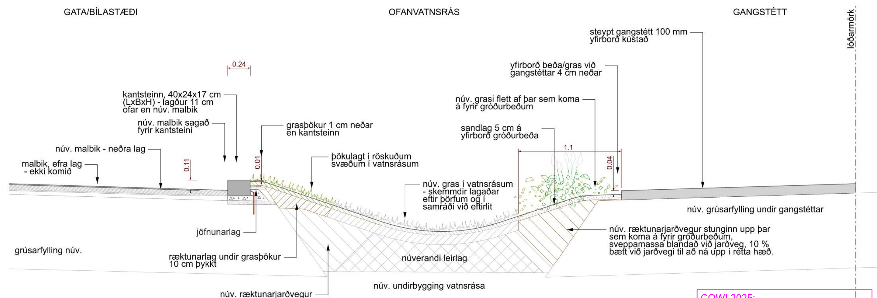
KENNISNIÐ B Mkv. 1:25 Kantur og gróðurbeð við götu og gangstétt
