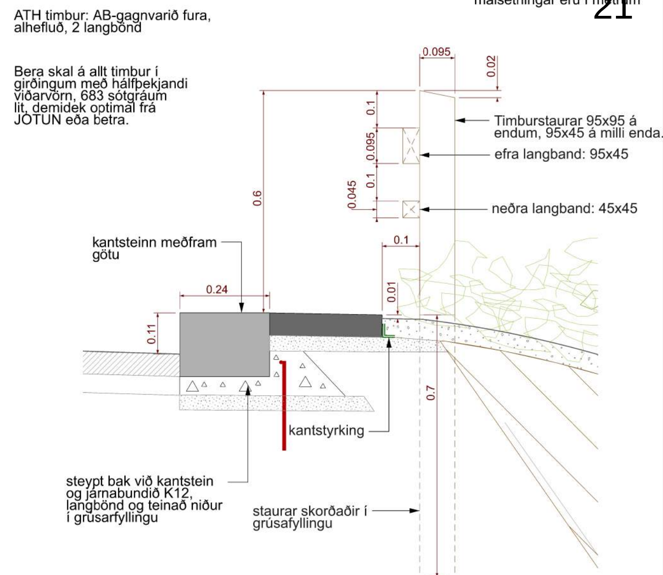
KENNISNIÐ A1 Mkv.1:10 Gróðurvarnargirðing og kantsteinn
