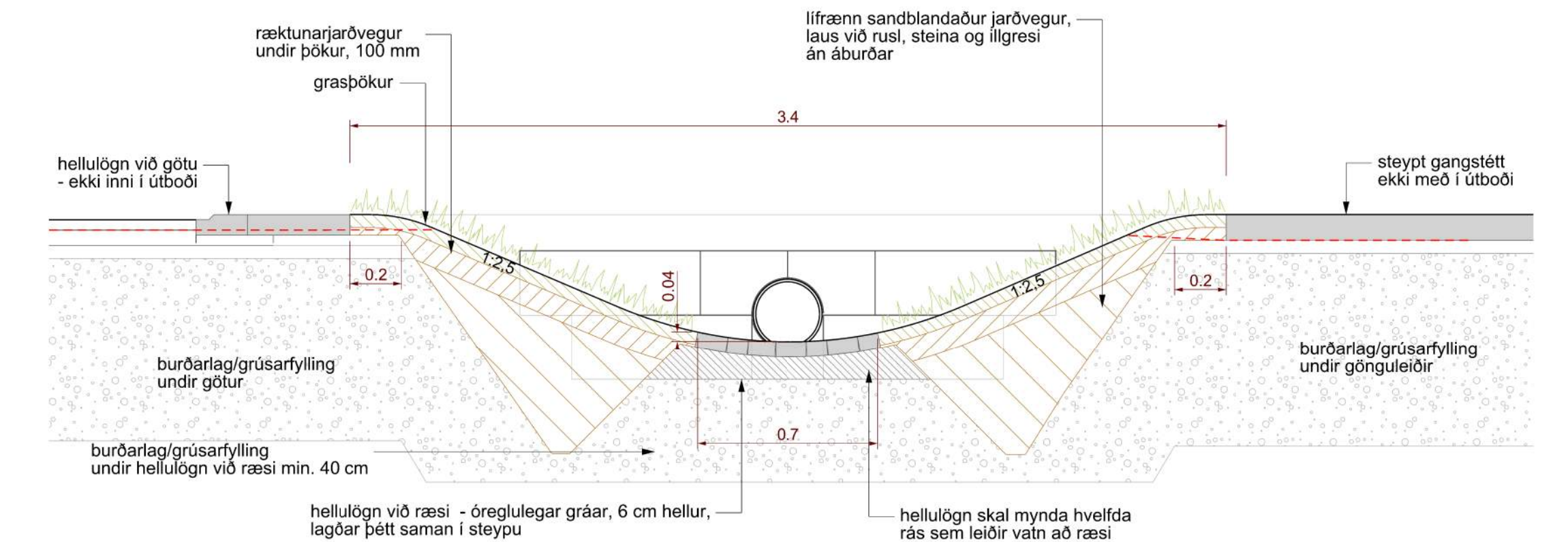
SNID C - þversnið og ásynd á frágang framan við grágrýtishleðslu, mkv. 1:20
