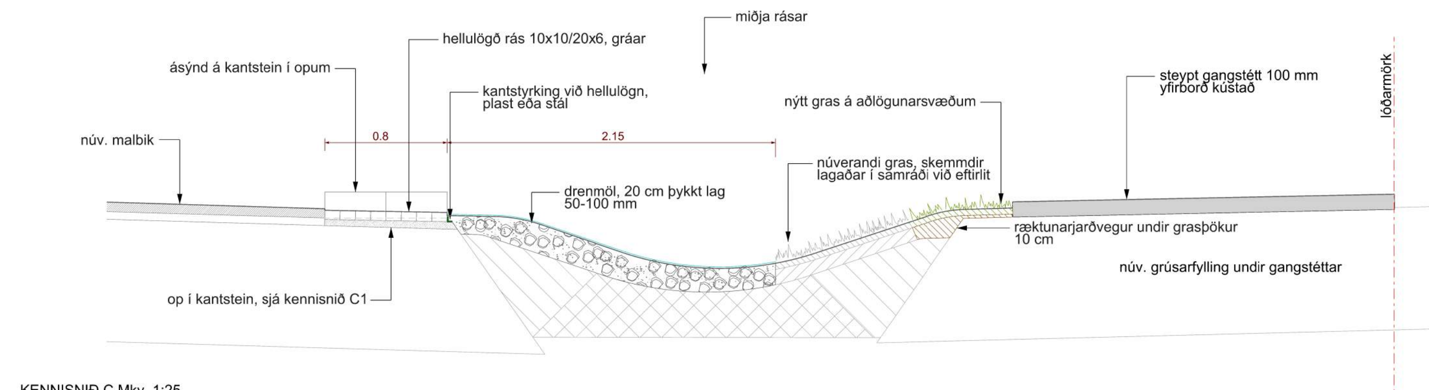
KENNISNIÐ C Mkv. 1:25 Op í kantstein og hellulögð rás
