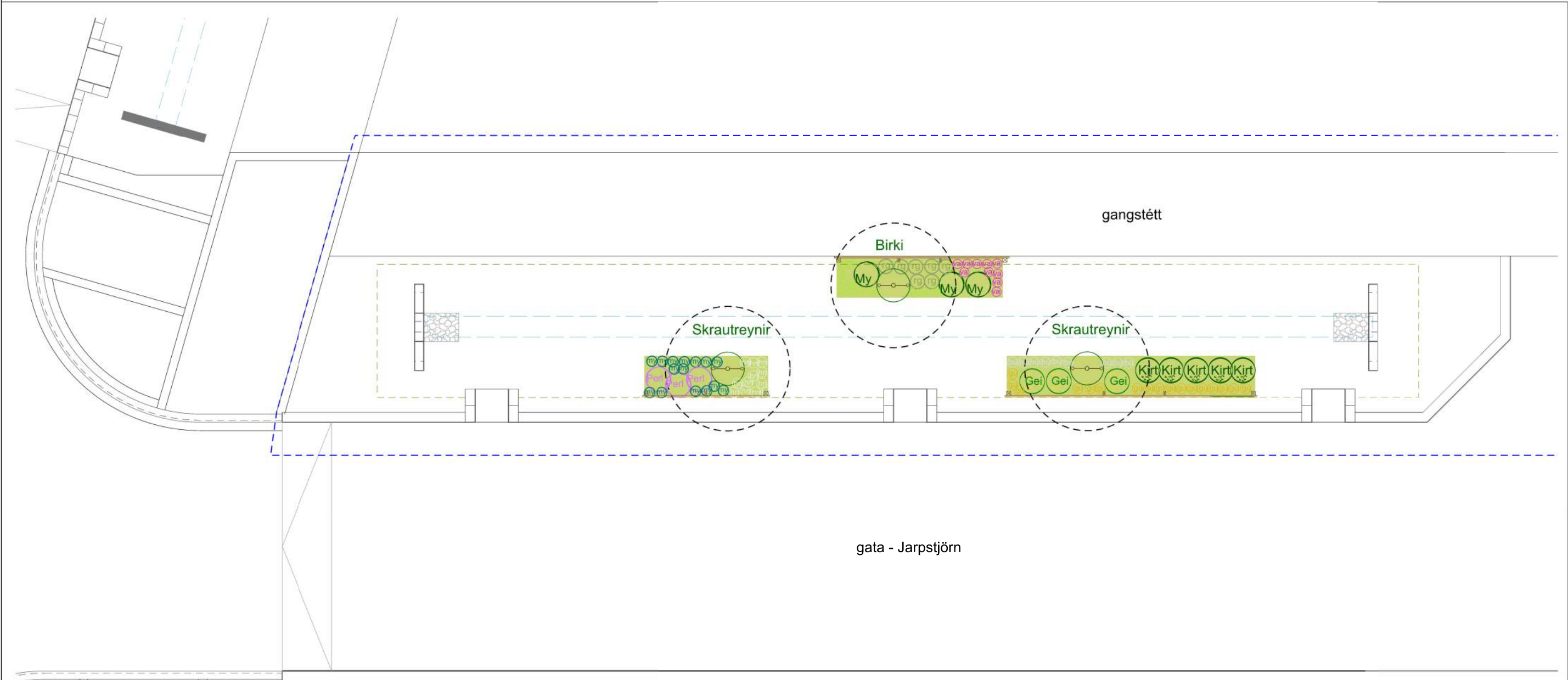
PLÖNTUPLAN Í VATNSRÁS SILFRATJÖRN 26-32 PLÖNTUPLAN GEFID ÚT Á VERKTÍMA
