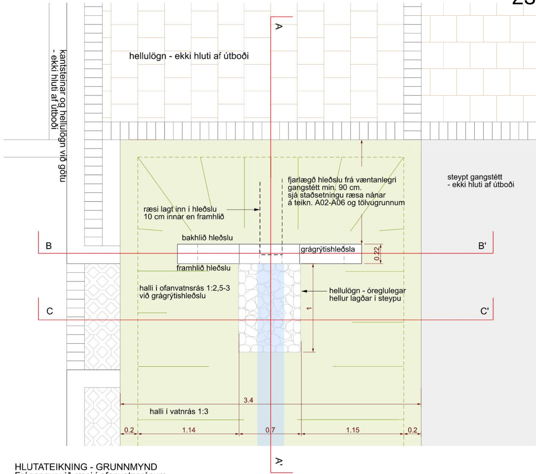
HLUTATEIKNING - GRUNNMYND Frágangur við ræsi í ofanvatnsrásum mkv. 1:25
