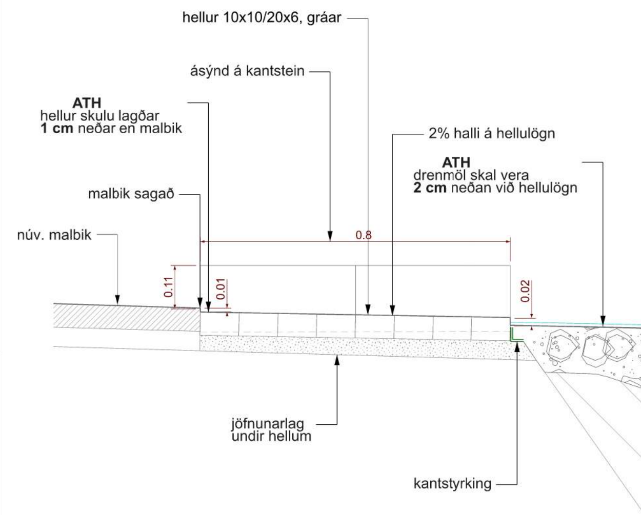
KENNISNIÐ C1 Mkv.1:10 Op í kantstein og hellulögð rás
