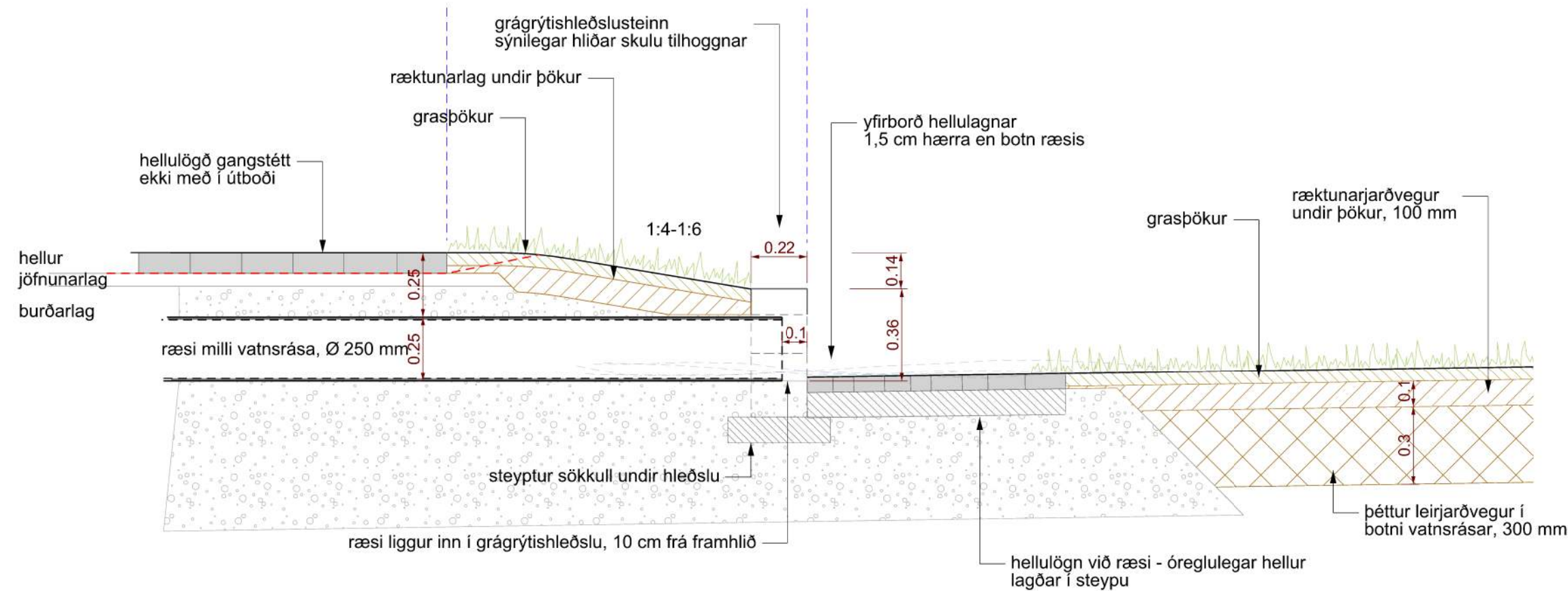
SNID A - langsnið í grágrýtishleðslu og ræsi, mkv. 1:20
