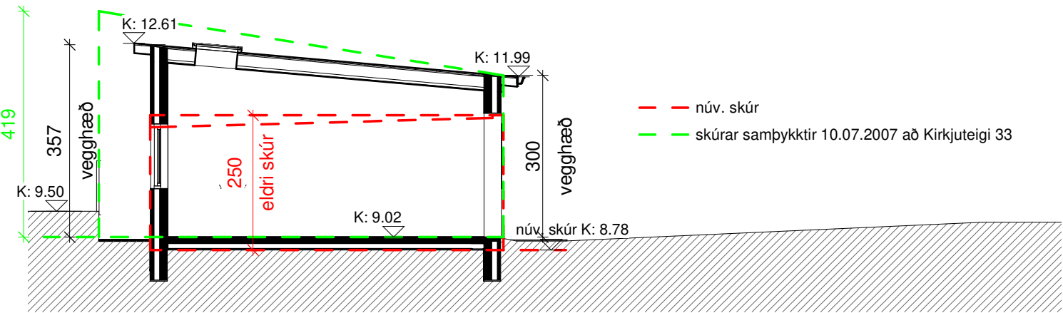
Þversnið í nýjan bílskúr/vinnustofu að Hraunteigi 30 1 : 100
