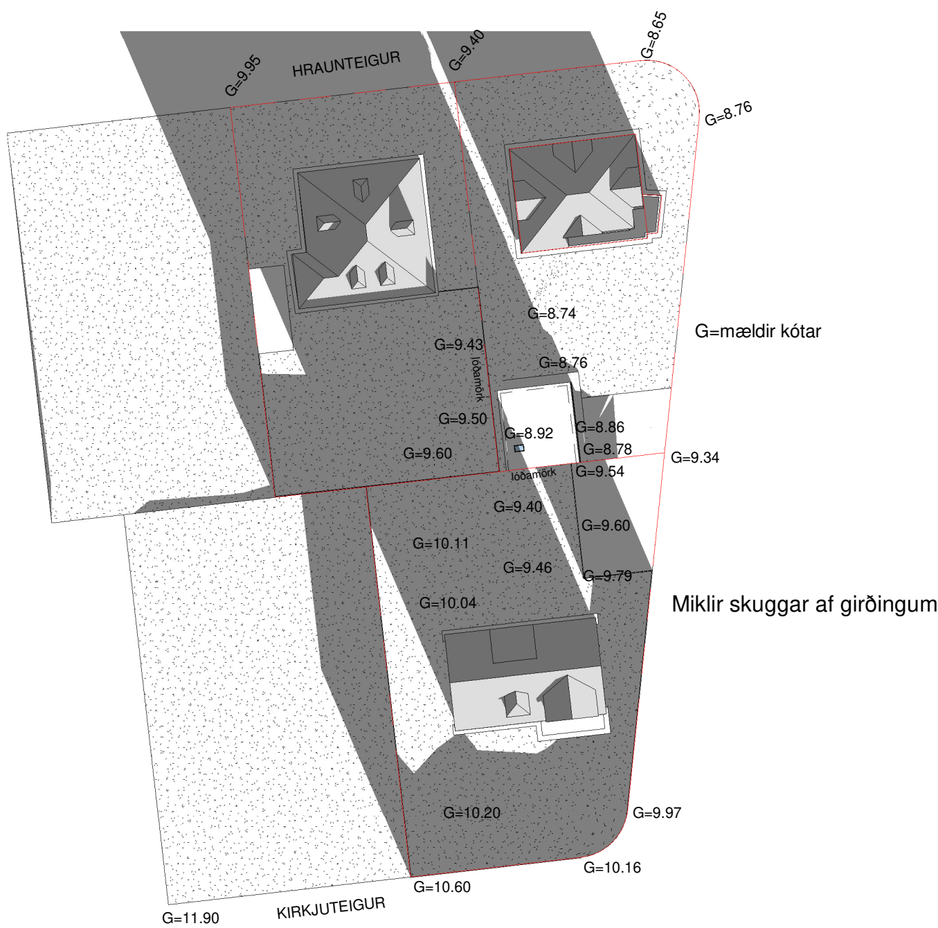
21. janúar kl.12 eftir breytingu 1 : 500
