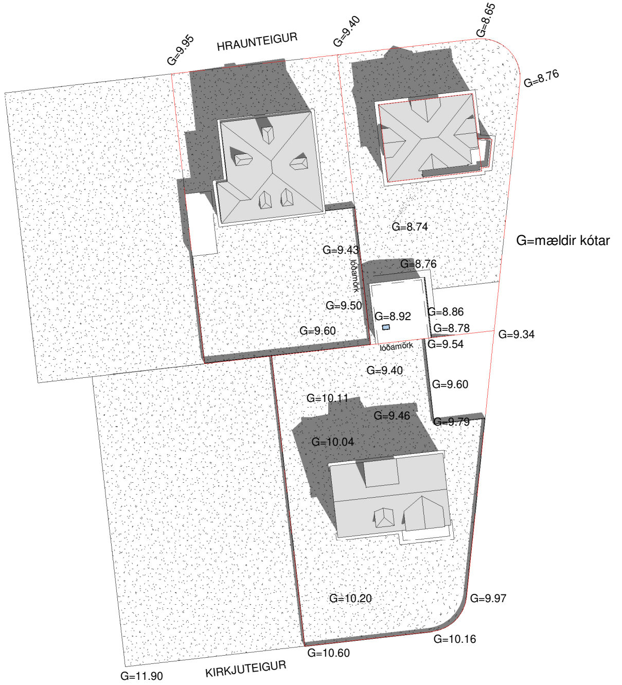
21. júní kl.12 eftir breytingu 1 : 500
