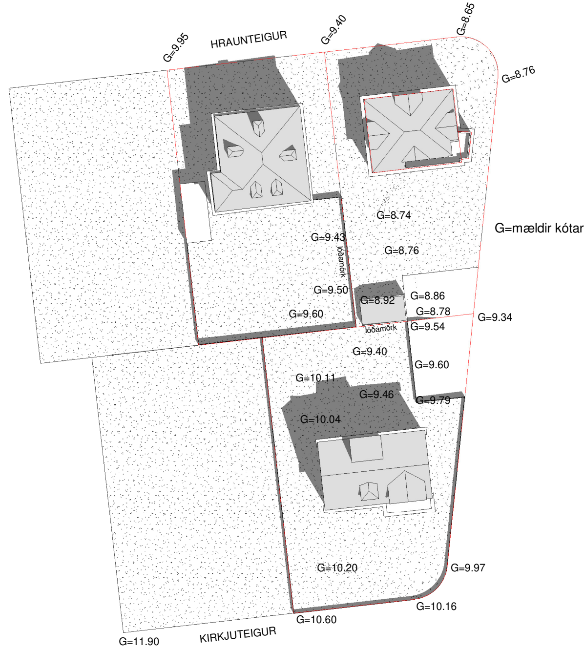
21. júní kl.12 fyrir breytingu 1 : 500
